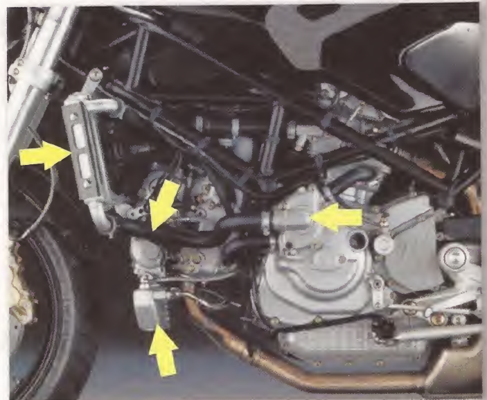
Refrigeración por líquido y aceite
